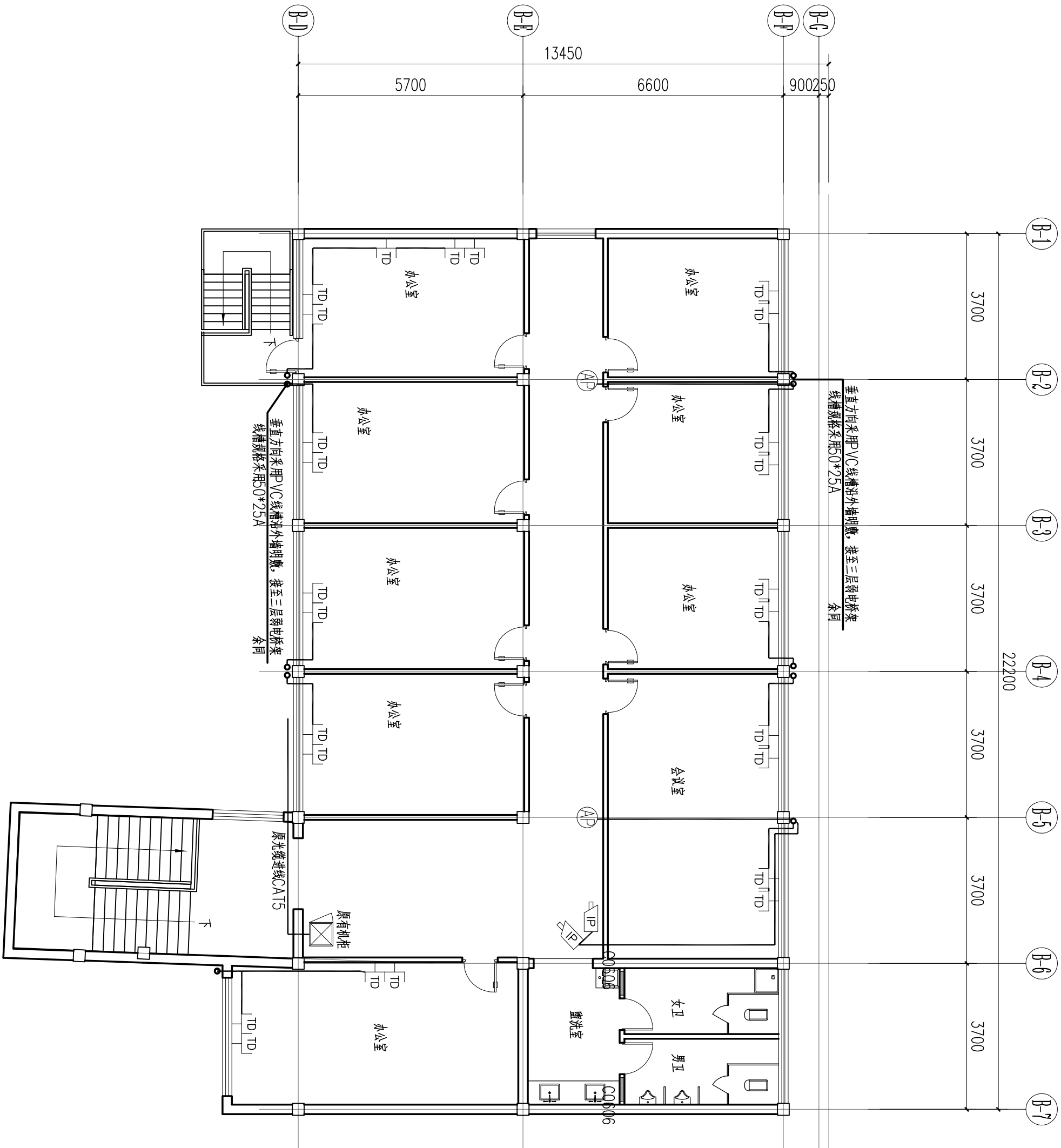
六层弱电平面图 1:100
